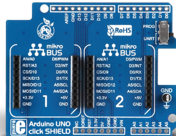
Arduino Uno Click Shield
